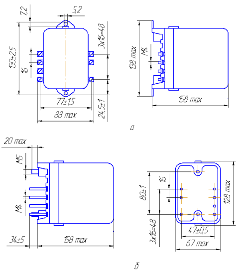
Рисунок 1 – Габаритные, установочные и присоединительные размеры реле типов РН-53, РН-54. Размеры без предельных отклонений – стандартные а – переднее присоединение б – заднее присоединение
